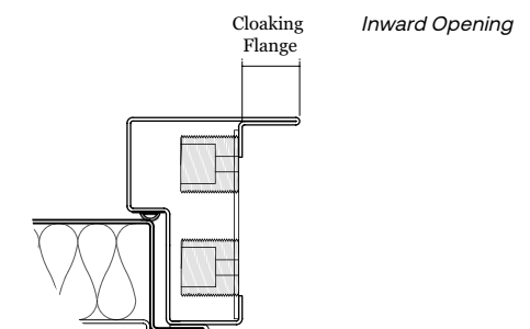
Inward Opening
